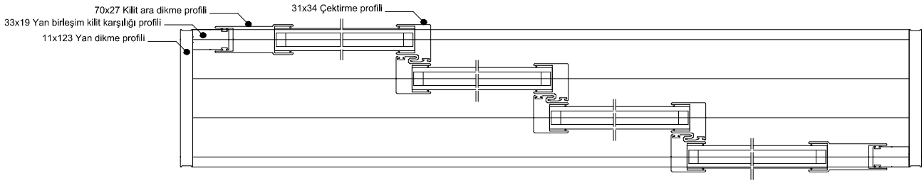
Slidemaster Twin / Üst görünüş
