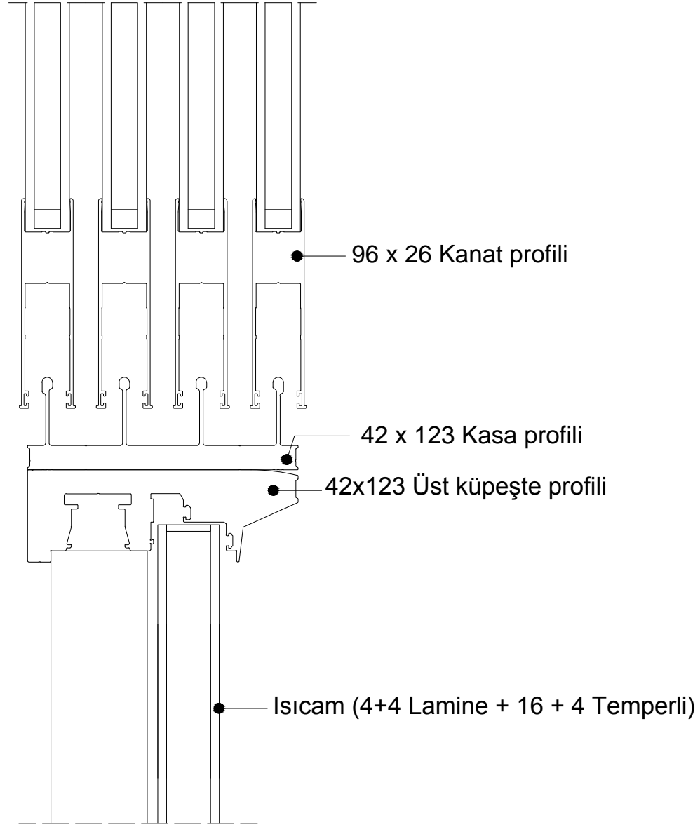
Slidemaster Twin + Balumax Twin Küpeşte
