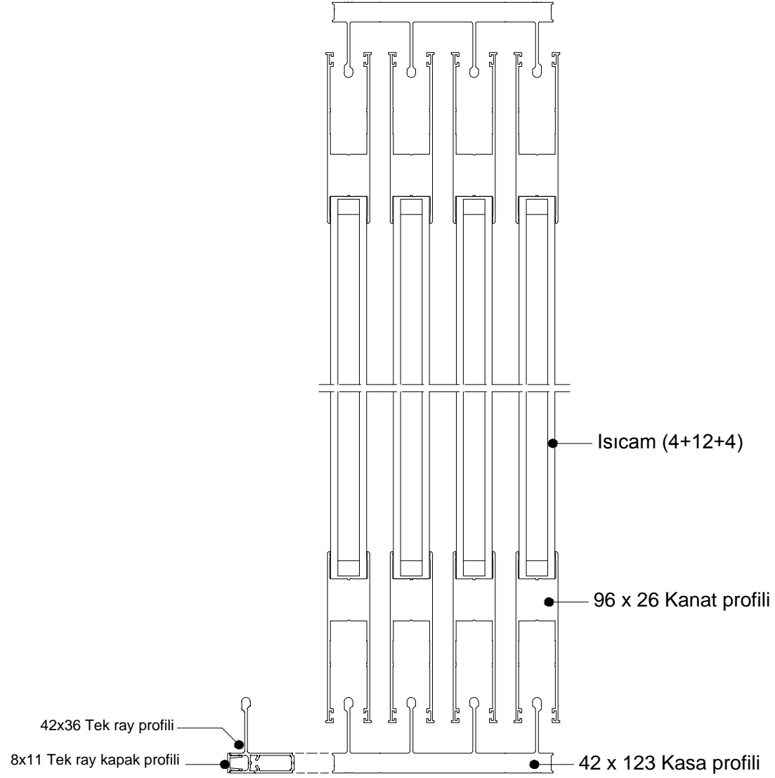
Slidemaster Twin / Yan görünüş
