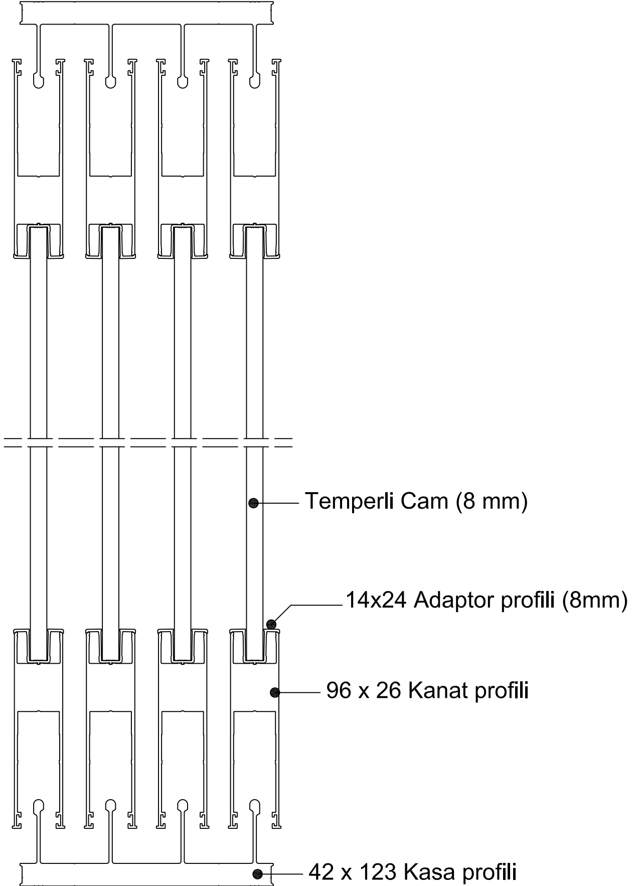
Slidemaster 08 / Yan görünüş
