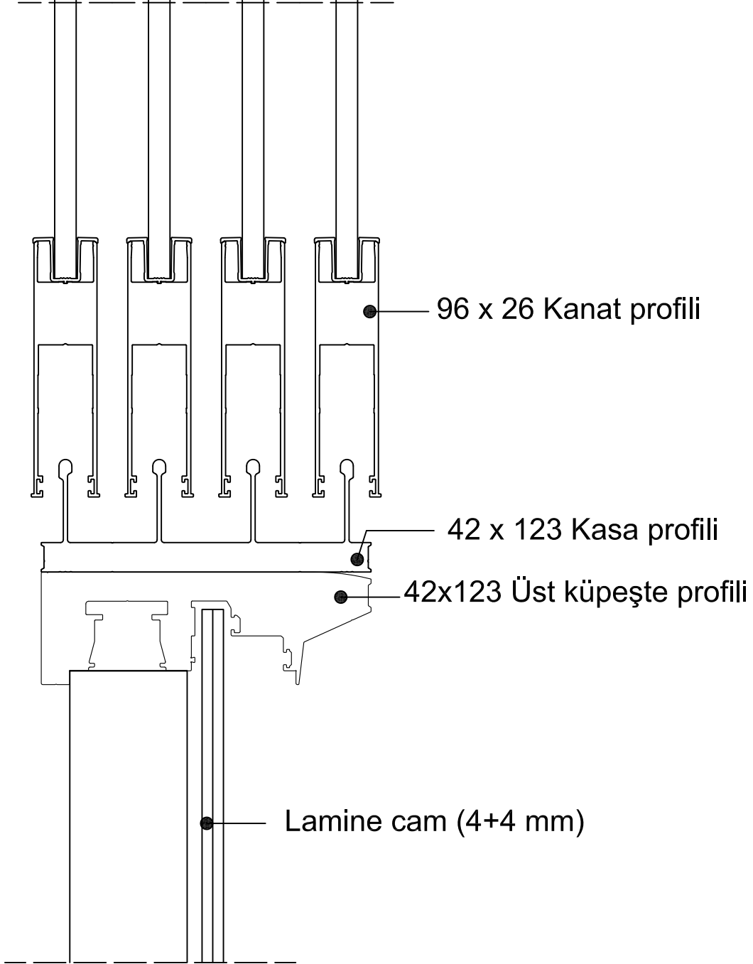
Slidemaster 08 + Balumax 08 Küpeşte
